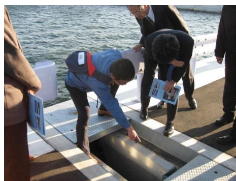
遮水構造の見学状況
